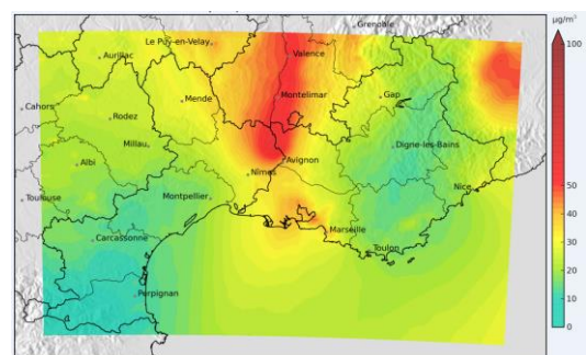
Moyenne journalière en PM10 le 21 mars 2016
