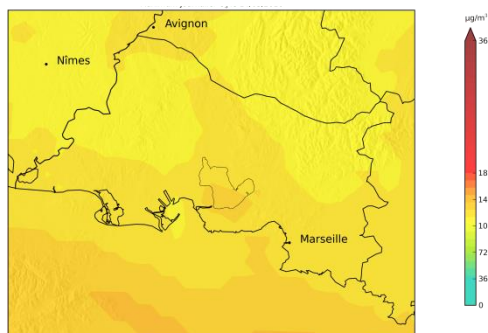
Maximum horaire en ozone le 14 mai 2016
