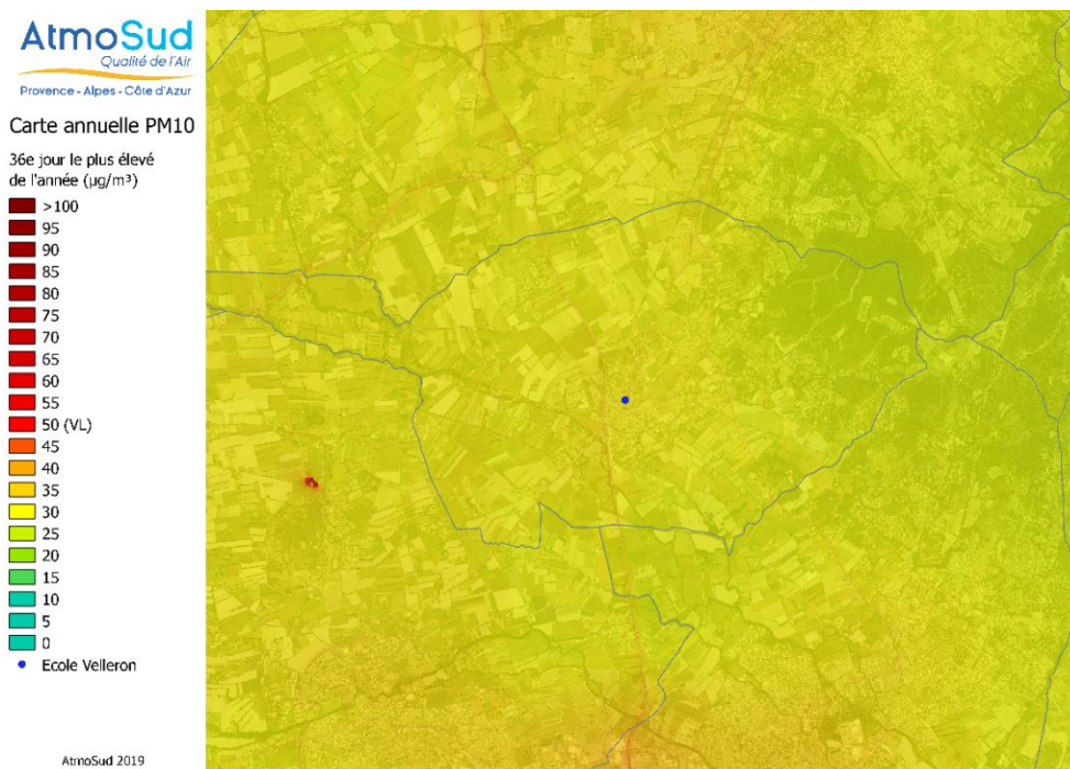
Figure 10 : Carte de pollution annuelle en PM 10 (2017)
