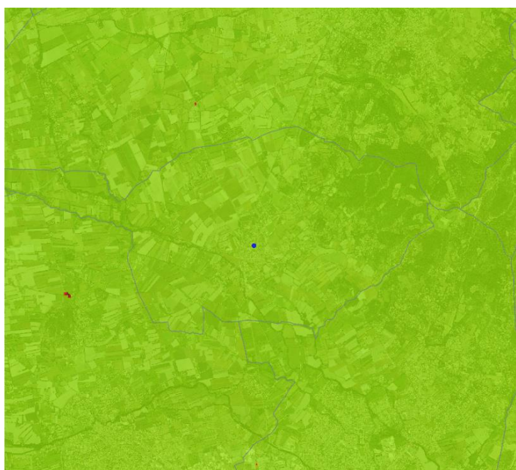
Figure 8 : Carte Stratégique Air (données 2017)
