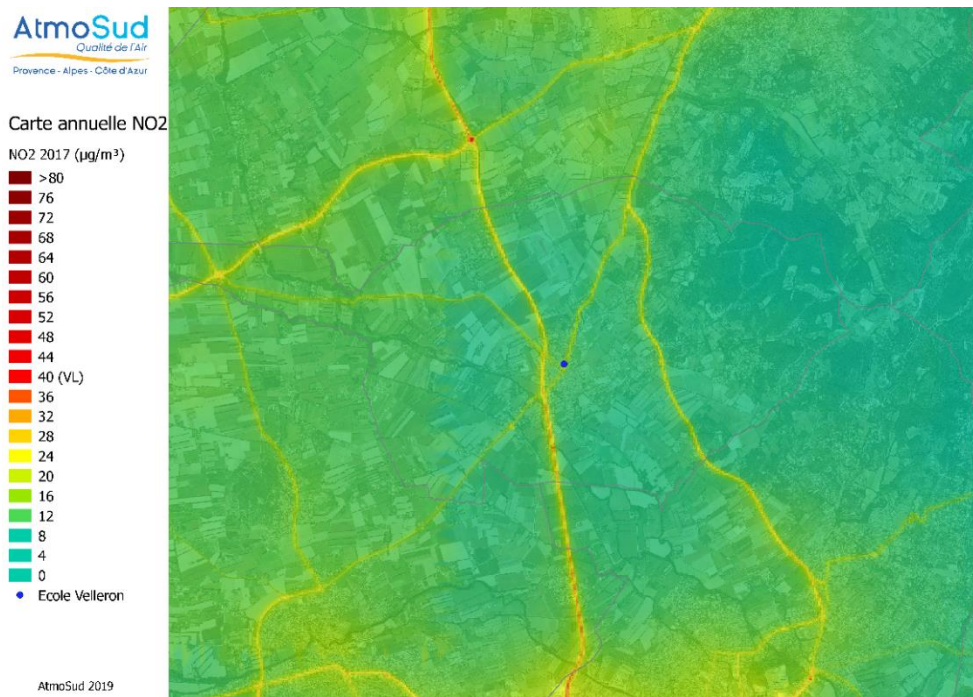
Figure 9 : Carte de pollution annuelle en dioxyde d'azote (2017)
