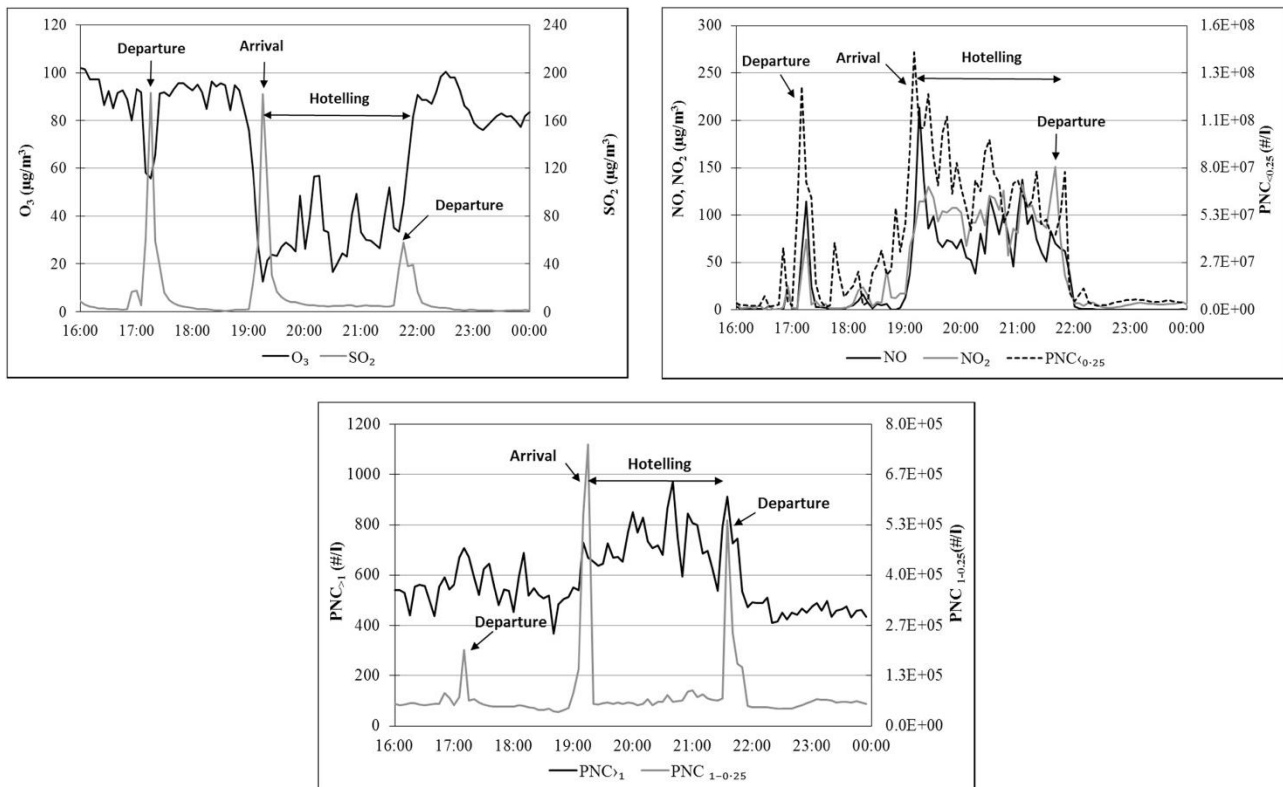
Figure 14 : Évolution des concentrations en polluants gazeux et en nombre de particules, dans différentes gammes de tailles, associées aux phases de manœuvre et de stationnement à quai (résolution : 5 min) (Merico et al., 2016)
