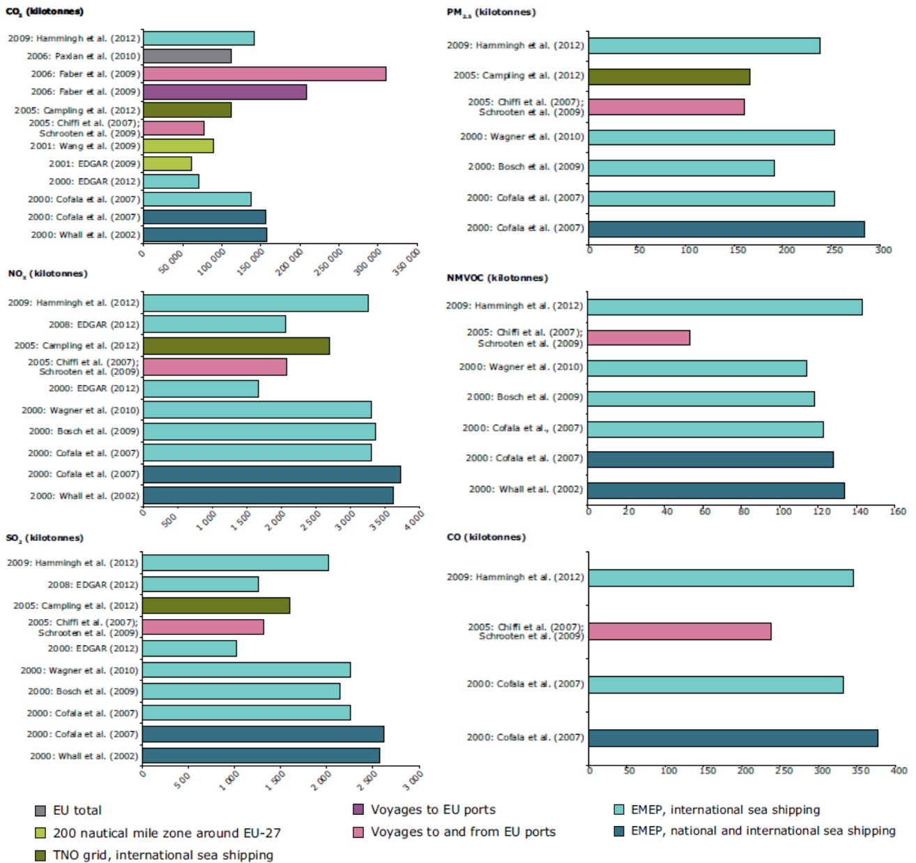
Figure 4 : Inventaires d'émissions des gaz à effet de serre et des polluants atmosphériques réalisés en Europe (EEA, 2013a)
