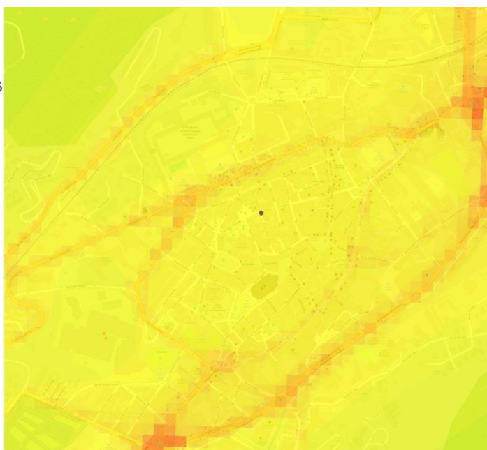
Figure 8 : Carte de pollution annuelle en PM10 (2016)
