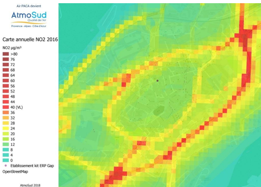
Figure 7 : Carte de pollution annuelle en dioxyde d'azote (2016)
