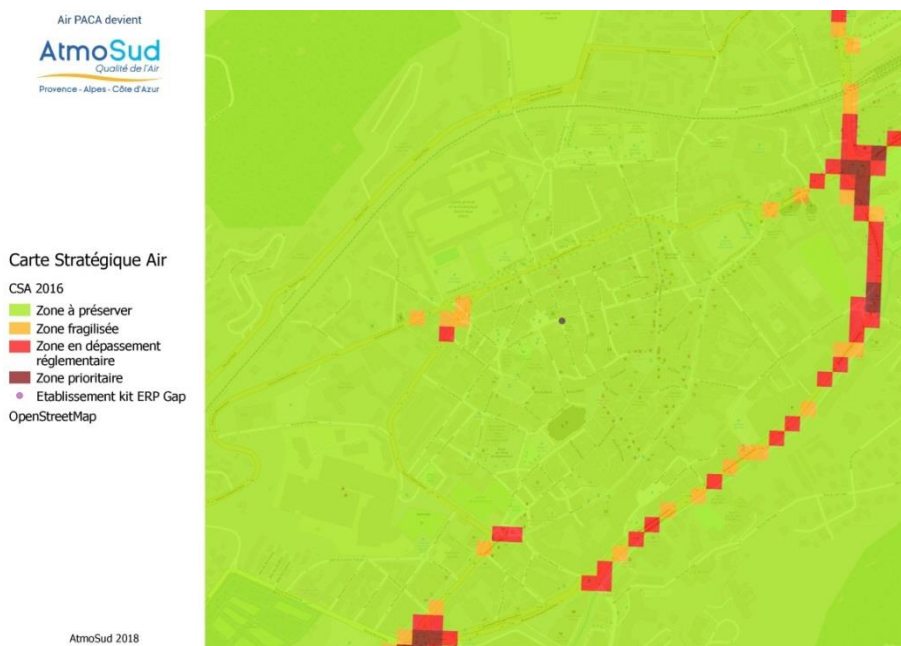
Figure 6 : Carte Stratégique Air (données 2016)
