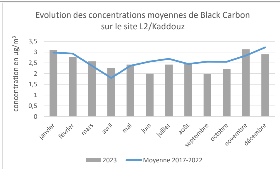
Figure 7 : Evolution du Black Carbon sur le site de Marseille / L2-Kaddouz en 2023
