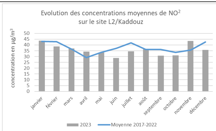
Figure 6 : Evolution du NO 2 sur le site de Marseille / L2-Kaddouz en 2023
