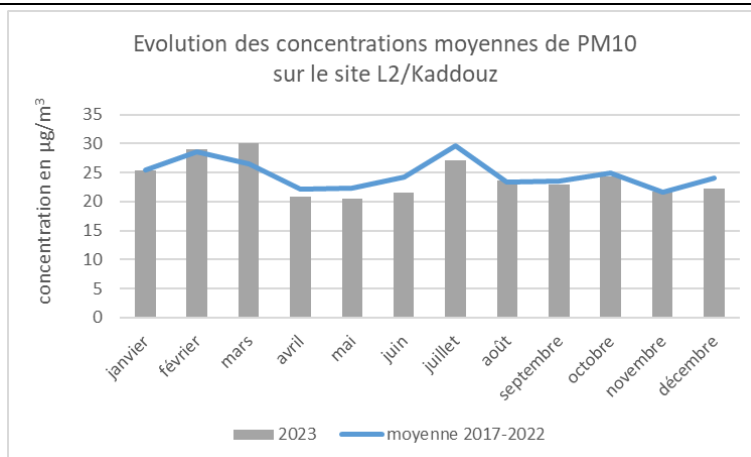
Figure 5 : Evolution des PM10 sur le site de Marseille / L2-Kaddouz en 2023
